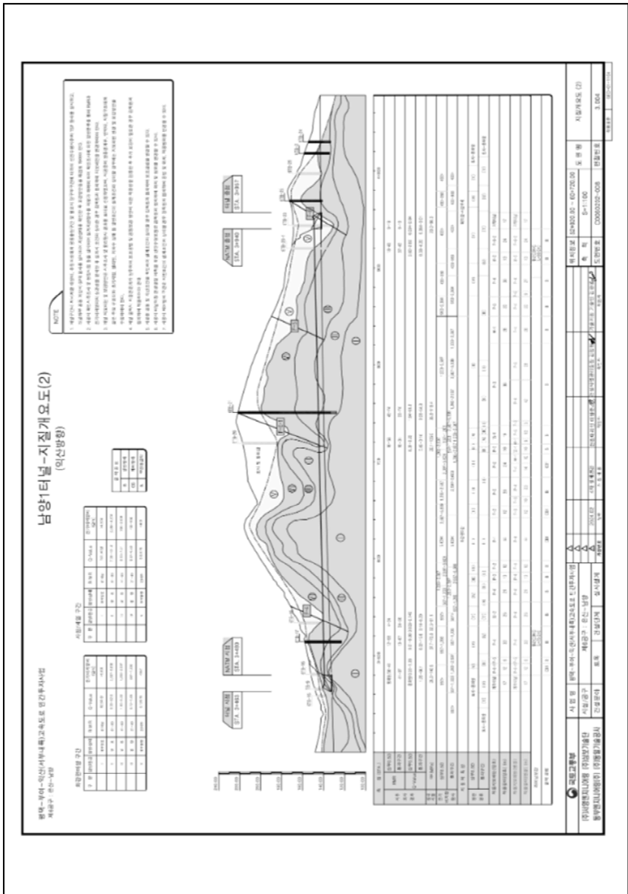
【그림 2.1.3】 지질개요도
